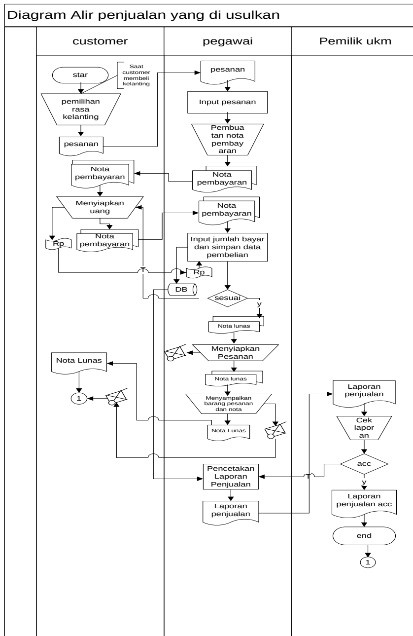
Gambar 3.2 Prosedur Transaksi yang diusulkan UKM kelanting khas telo
