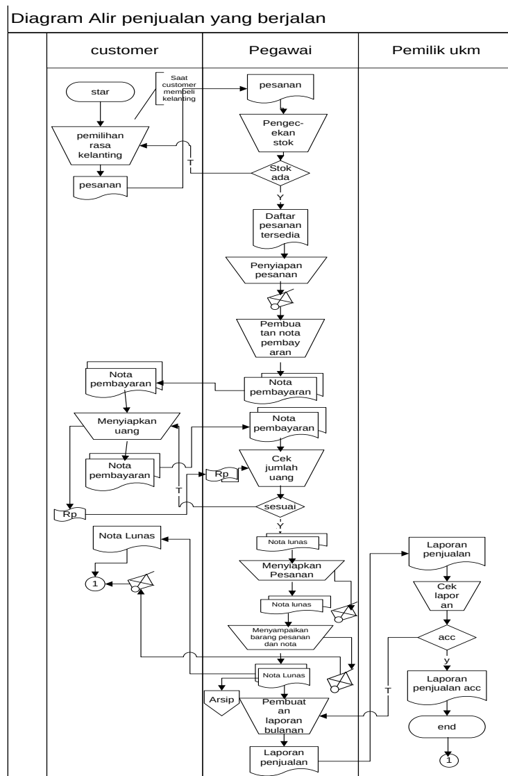
Gambar 3.1 Prosedur Transaksi berjalan UKM kelanting khas telo
