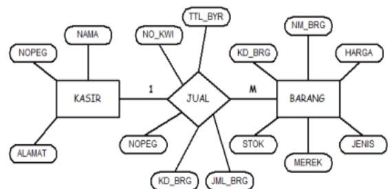
Gambar 3.9 Rancangan ERD.
