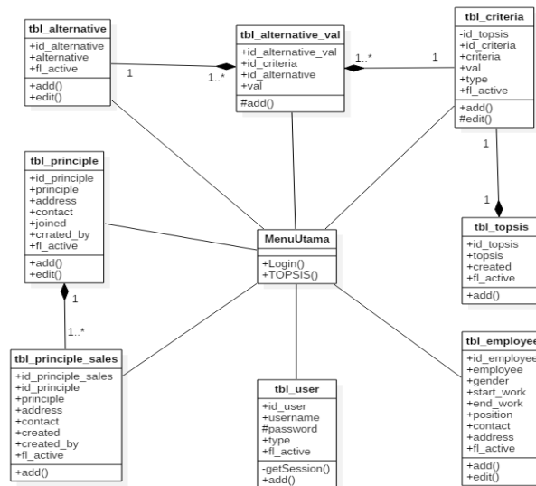
Gambar 3. Class Diagram Sistem Yang Diusulkan
