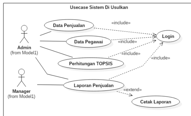
Gambar 2. Sistem Use Case Admin Yang Diusulkan
