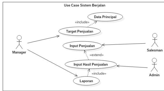
Gambar 1. Use Case Sistem Yang Berjalan
