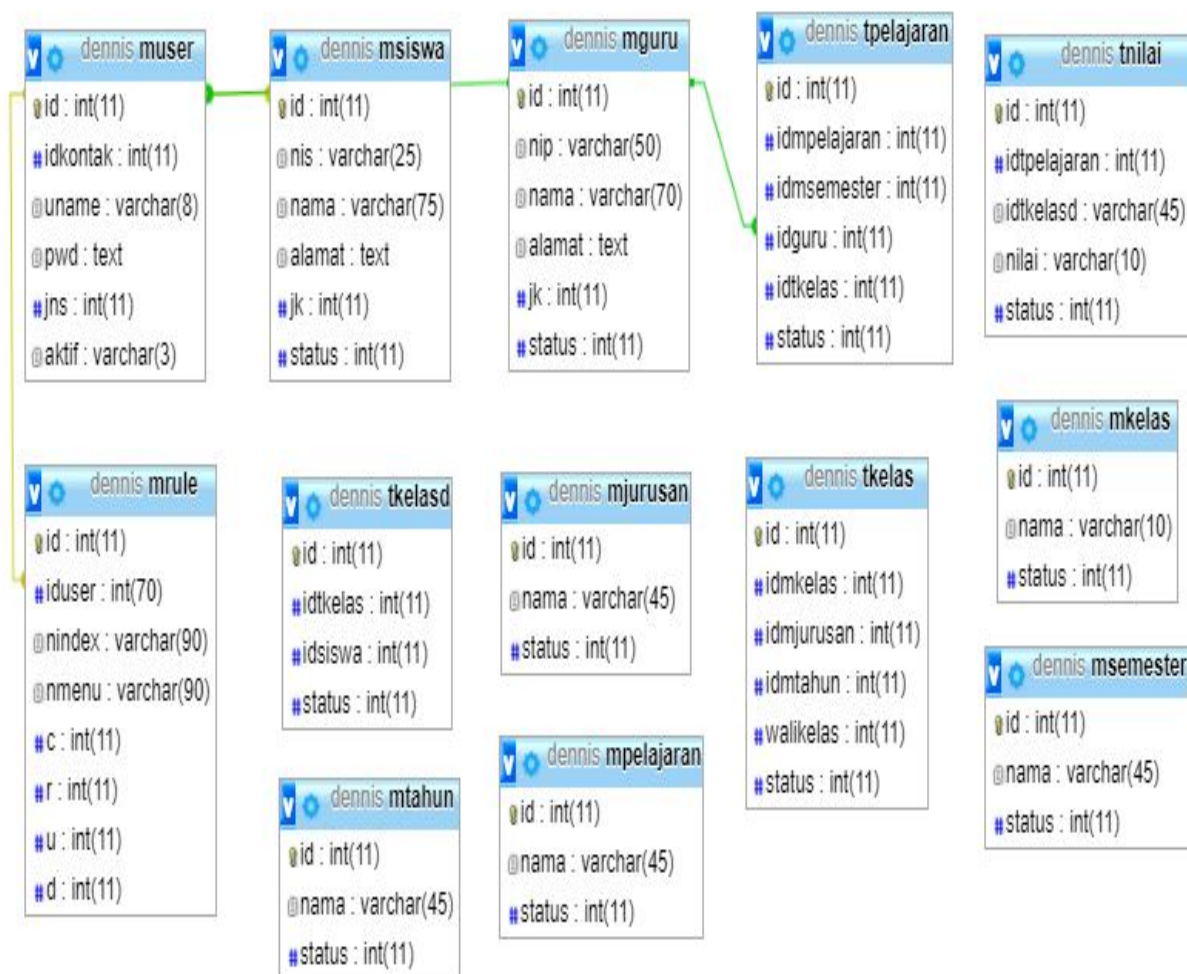
Gambar 2.4.Relasi Antar Table
