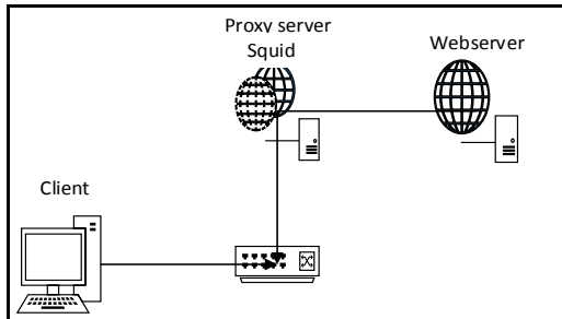
Gambar 1. Skema Pengujian 1
